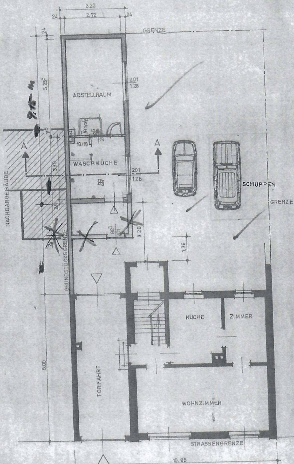
GRUNDRISS
